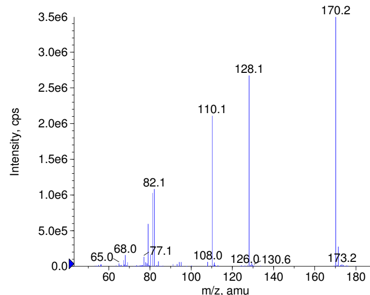
+ Aceclidine Prec(170.0) CE(99.0) RT(0.8)
