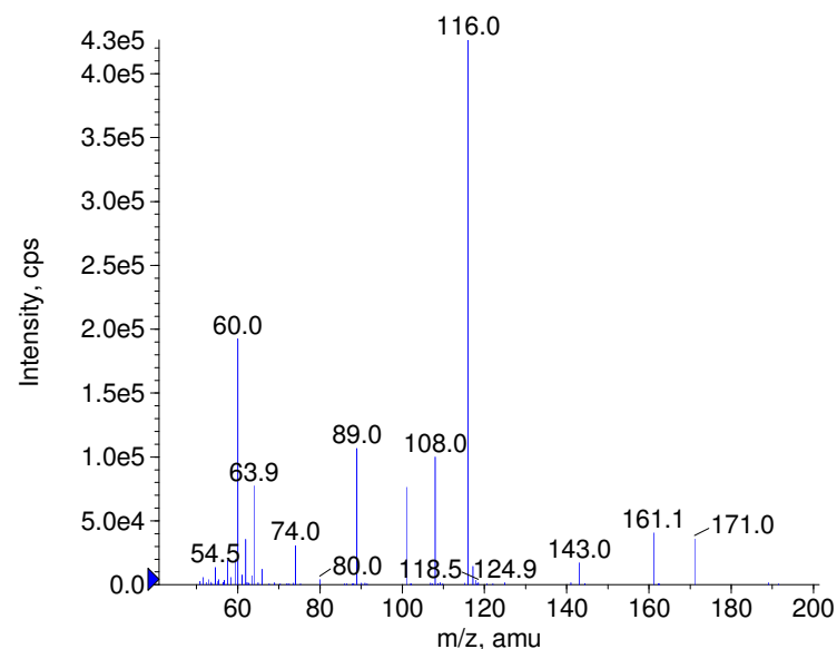
+ Amiloride Prec(230.0) CE(50.0) RT(0.8)
