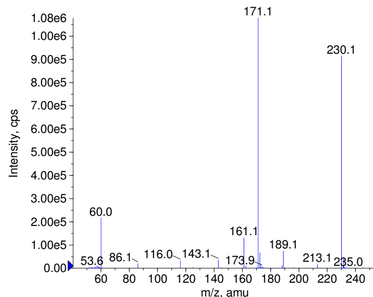
+ Amiloride Prec(230.0) CE(50.0) RT(0.8)
