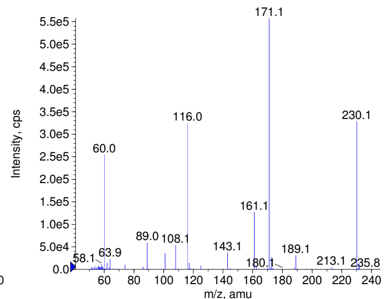
+ Amiloride Prec(230.0) CE(99.0) RT(0.8)
