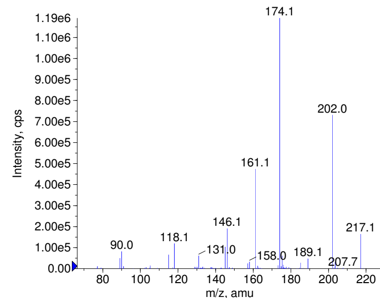
+ Ammoidin Prec(217.0) CE(99.0) RT(1.1)
