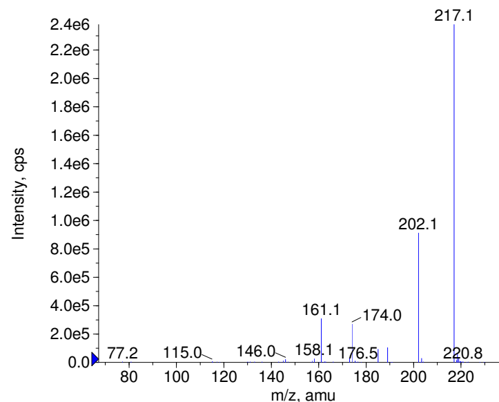
+ Ammoidin Prec(217.0) CE(50.0) RT(1.1)
