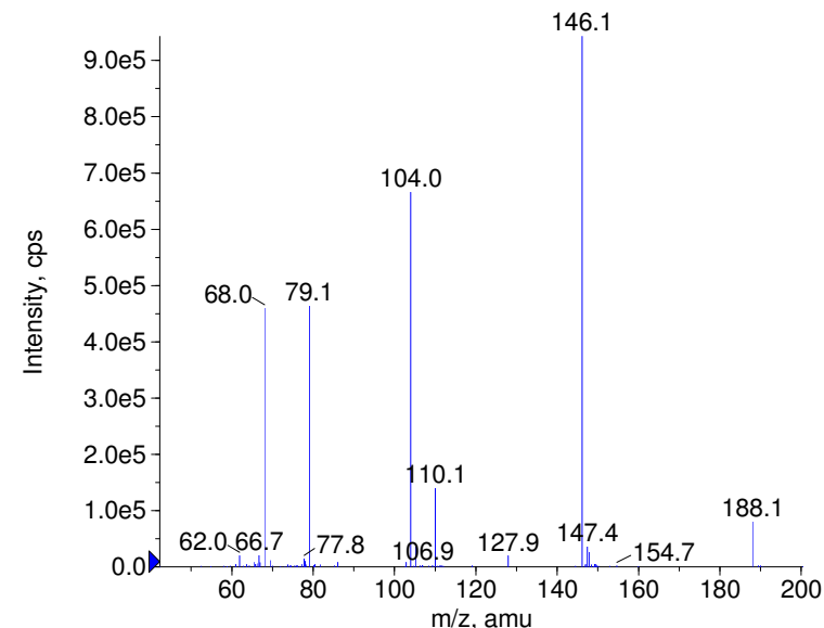
+ Atrazine-desethyl Prec(188.0) CE(99.0) RT(1.0)
