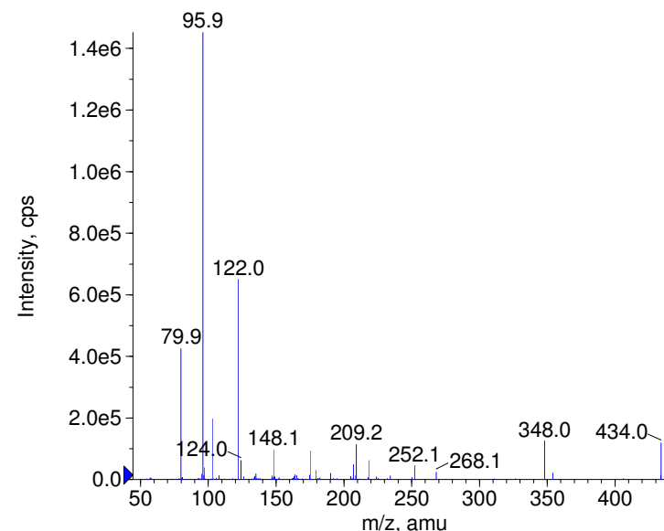
■ - Aztreonam Prec(434.0) CE(-99.0) RT(0.9)
