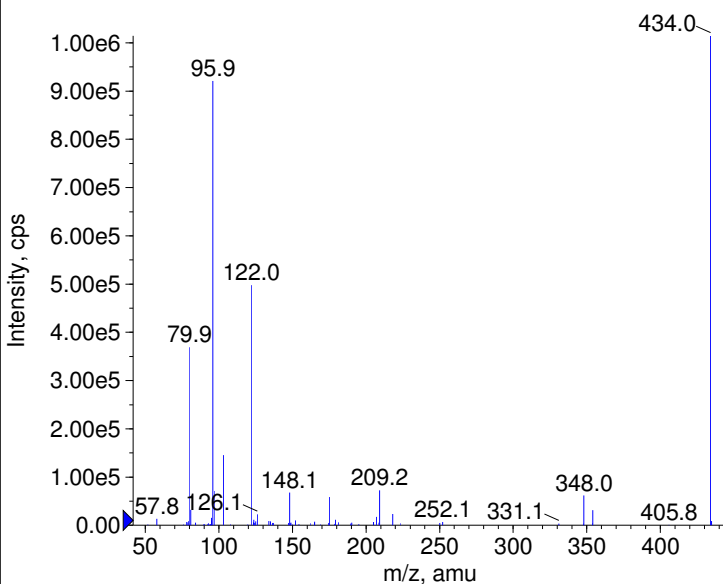
■ - Aztreonam Prec(434.0) CE(-99.0) RT(0.9)
