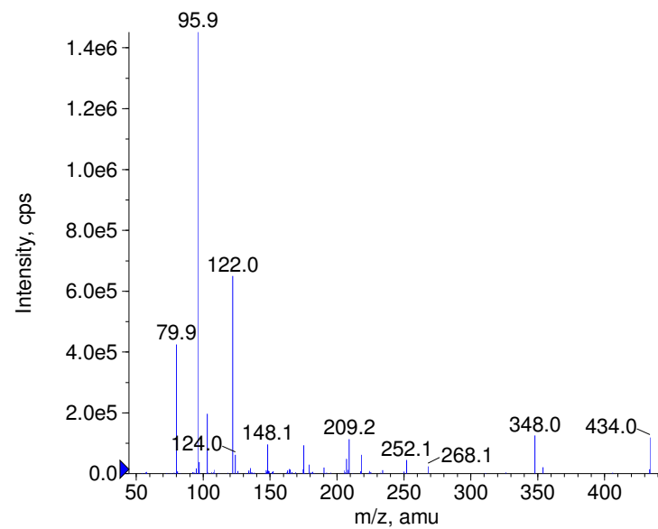
■ - Aztreonam Prec(434.0) CE(-35.0) RT(0.9)
