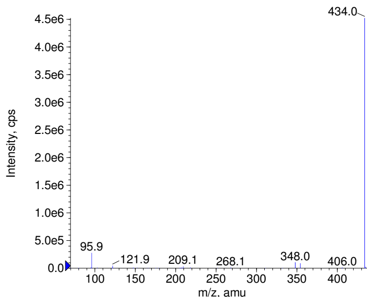
■ - Aztreonam Prec(434.0) CE(-50.0) RT(0.9)
