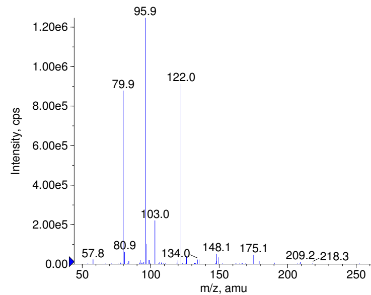
■ - Aztreonam Prec(434.0) CE(-50.0) RT(0.9)
