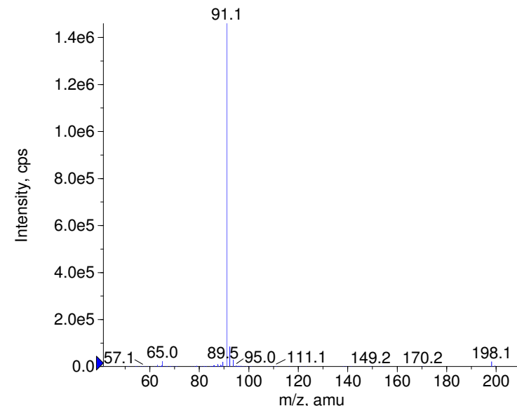
+ Beclamide Prec(198.0) CE(99.0) RT(1.2)
