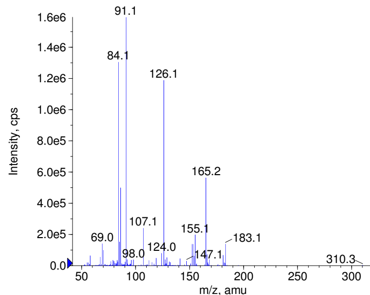
+ Benproperine Prec(310.0) CE(50.0) RT(0.9)
