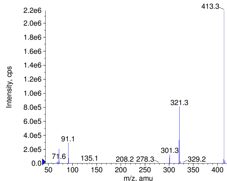
■ + Benzethonium Prec(413.0) CE(99.0) RT(4.1)
