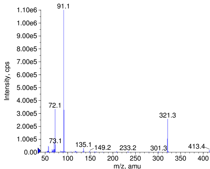
■ + Benzethonium Prec(413.0) CE(50.0) RT(4.1)
