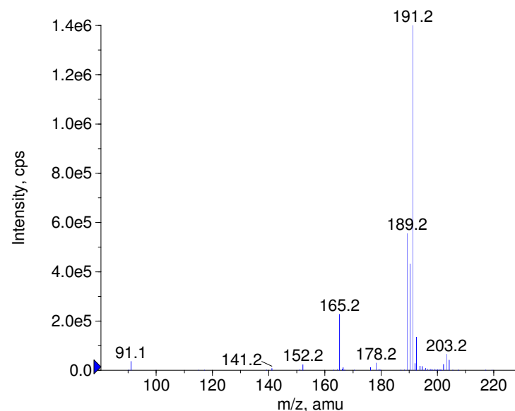
+ Benzoctamine Prec(250.0) CE(50.0) RT(0.8)
