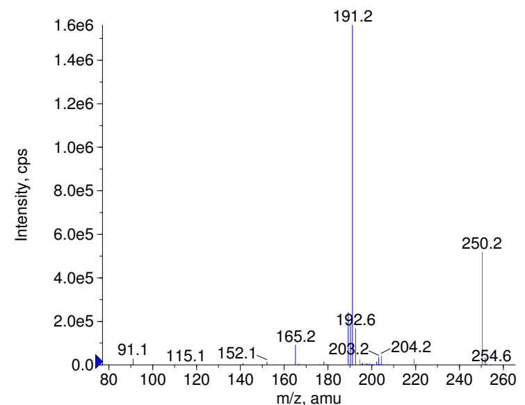
+ Benzoctamine Prec(250.0) CE(99.0) RT(0.8)
