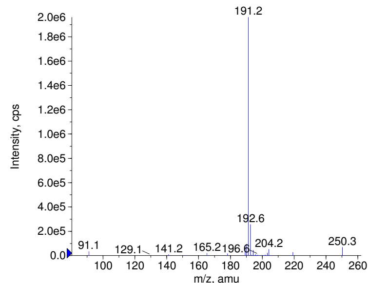
+ Benzoctamine Prec(250.0) CE(99.0) RT(0.8)
