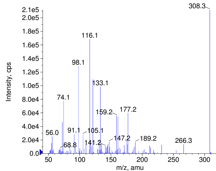
+ Betaxolol Prec(308.0) CE(99.0) RT(0.7)
