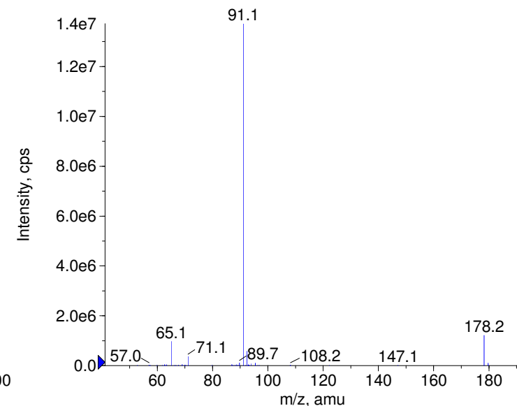
+ Bethanidine Prec(178.0) CE(99.0) RT(0.9)
