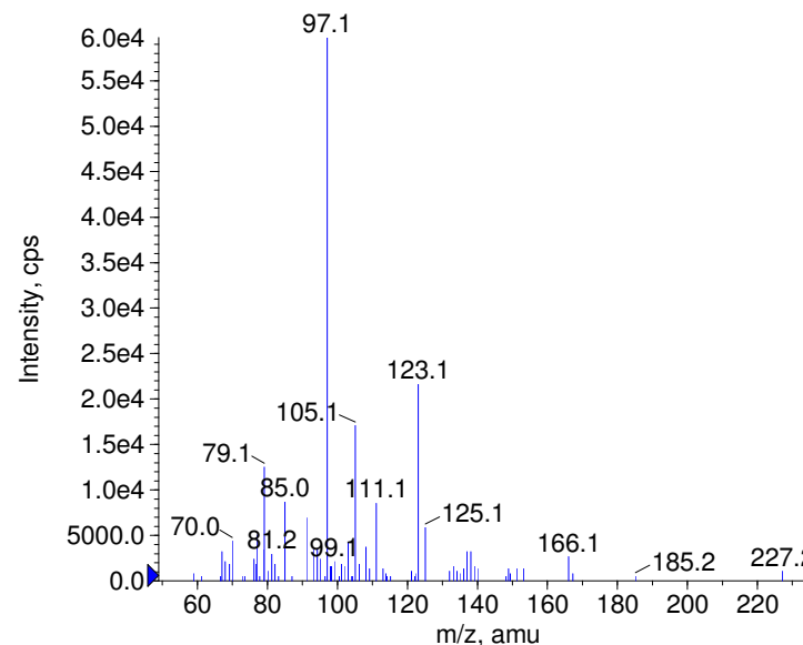
+ Biotin Prec(245.0) CE(50.0) RT(0.8)
