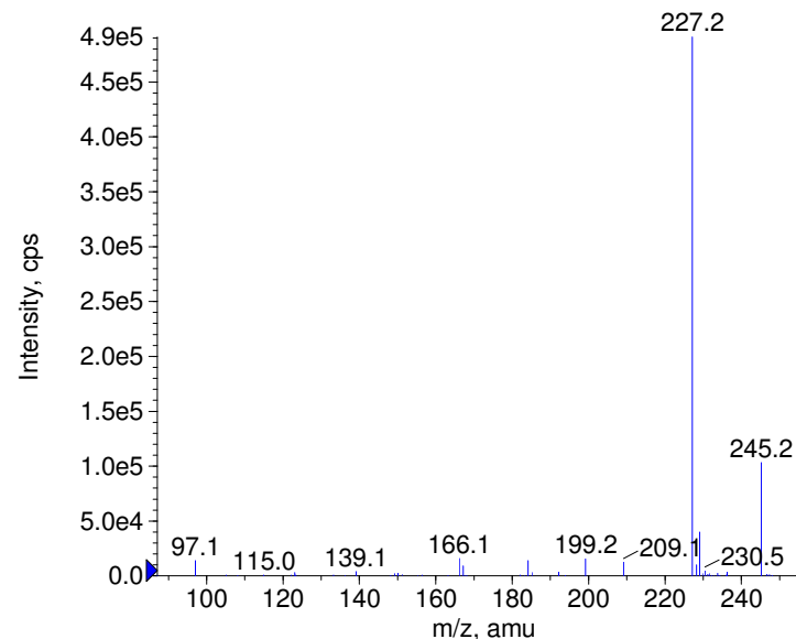
+ Biotin Prec(245.0) CE(50.0) RT(0.8)
