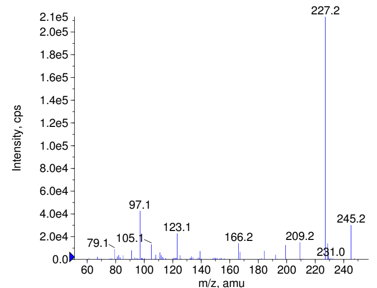
+ Biotin Prec(245.0) CE(99.0) RT(0.8)
