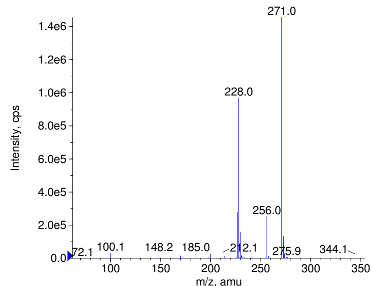
+ Bromopride Prec(344.0) CE(99.0) RT(0.9)
