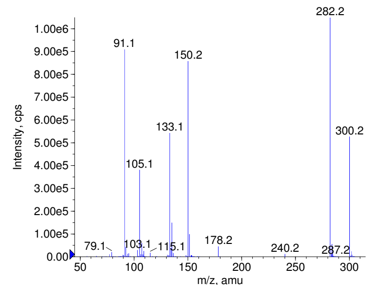
+ Buphenine Prec(300.0) CE(99.0) RT(0.9)
