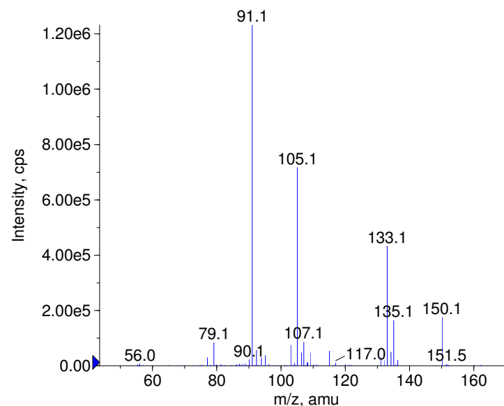
+ Buphenine Prec(300.0) CE(50.0) RT(0.9)
