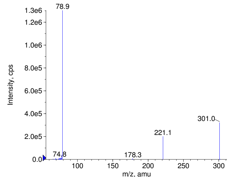
■ - Butallylonal Prec(301.0) CE(-99.0) RT(1.1)
