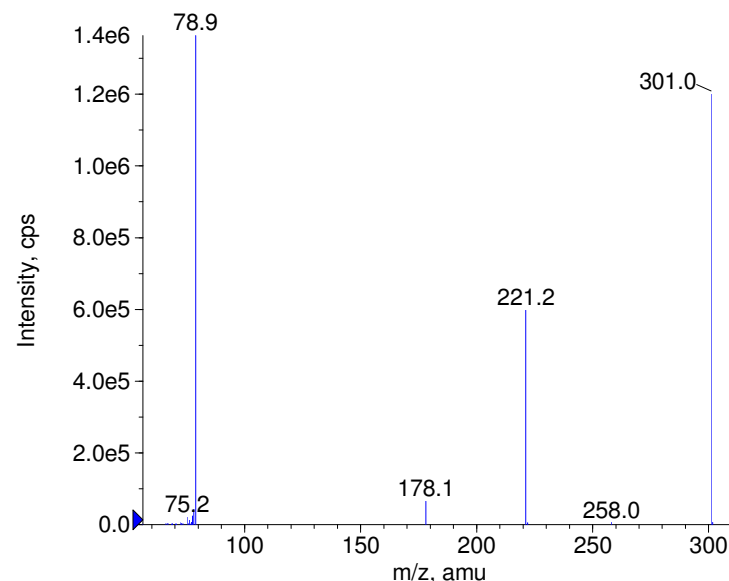
■ - Butallylonal Prec(301.0) CE(-50.0) RT(1.1)
