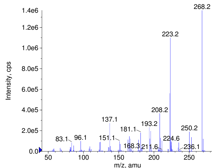
+ Cafaminol Prec(268.0) CE(99.0) RT(0.8)
