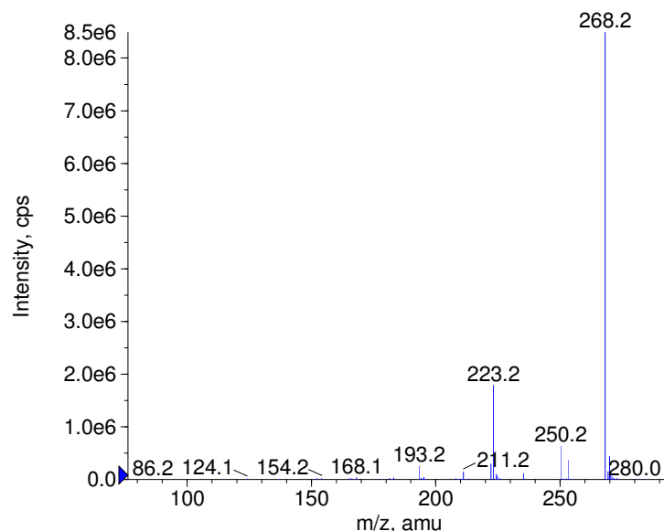
+ Cafaminol Prec(268.0) CE(50.0) RT(0.8)
