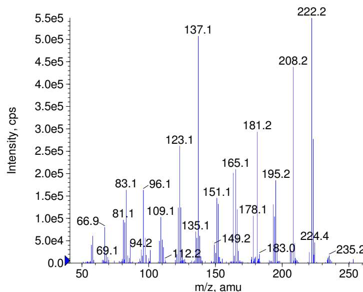
+ Cafaminol Prec(268.0) CE(50.0) RT(0.8)
