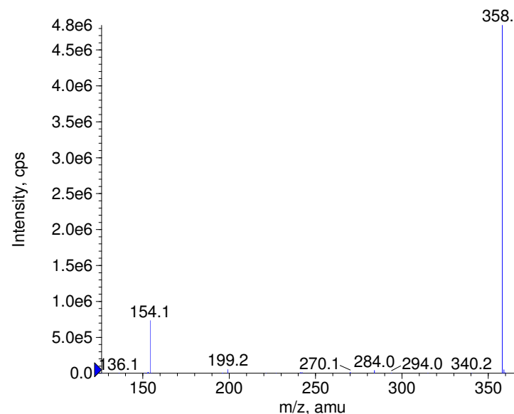
■ - Capecitabine Prec(358.0) CE(-50.0) RT(0.9)
