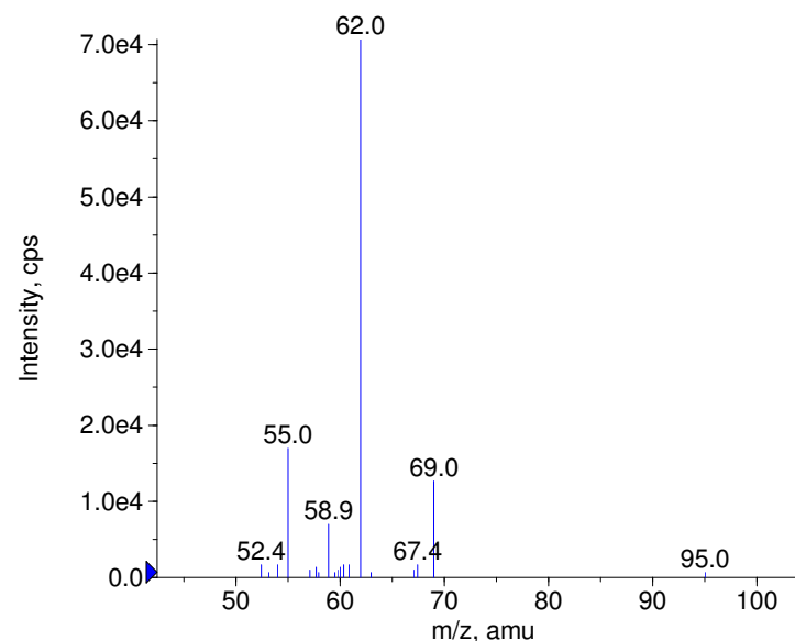
■ + Carisoprodol Prec(261.0) CE(50.0) RT(0.8)
