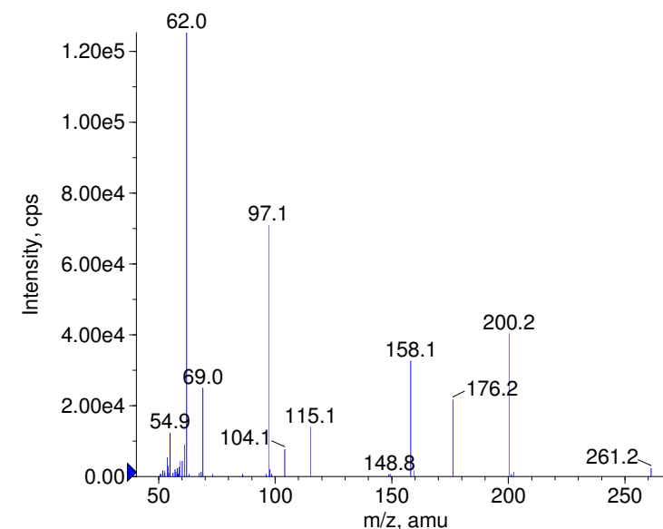
■ + Carisoprodol Prec(261.0) CE(99.0) RT(0.8)
