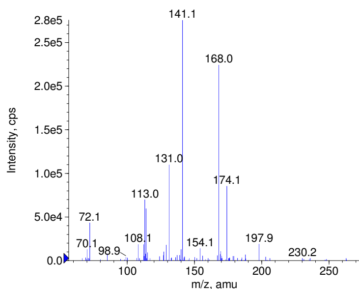
+ Cefotiam Prec(526.0) CE(50.0) RT(1.0)
