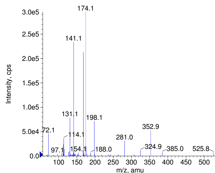
+ Cefotiam Prec(526.0) CE(99.0) RT(1.0)
