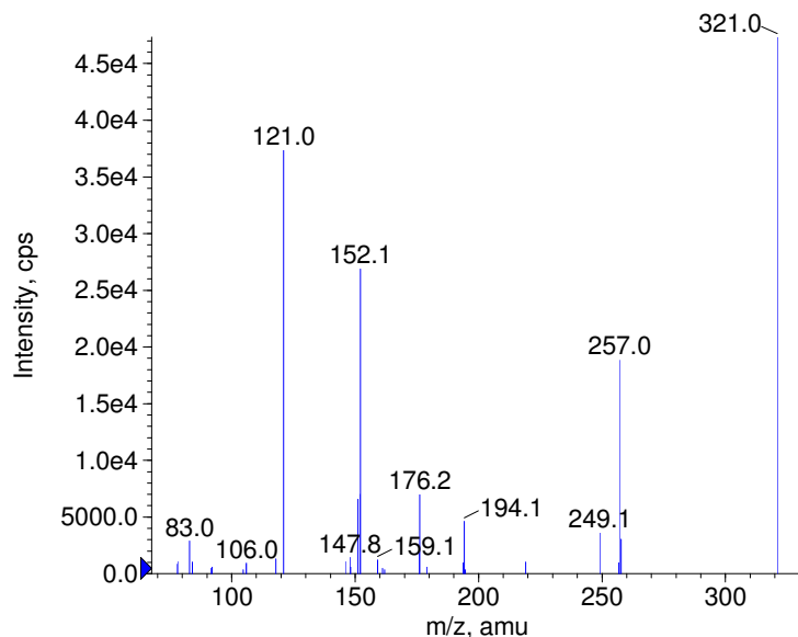
■ - Chloramphenicol Prec(321.0) CE(-99.0) RT(0.9)
