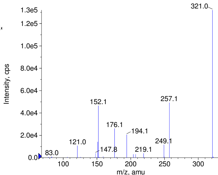
■ - Chloramphenicol Prec(321.0) CE(-50.0) RT(0.9)
