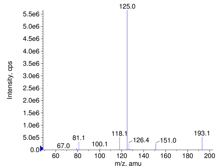
+ Chlorphencyclan Prec(310.0) CE(99.0) RT(1.0)
