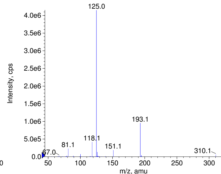
+ Chlorphencyclan Prec(310.0) CE(99.0) RT(1.0)
