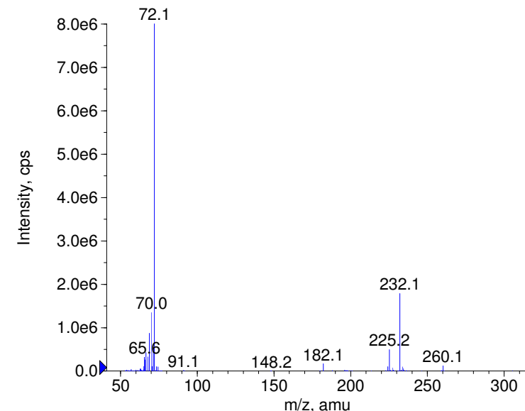
+ Chlorphenethiazine Prec(305.0) CE(99.0) RT(0.9)
