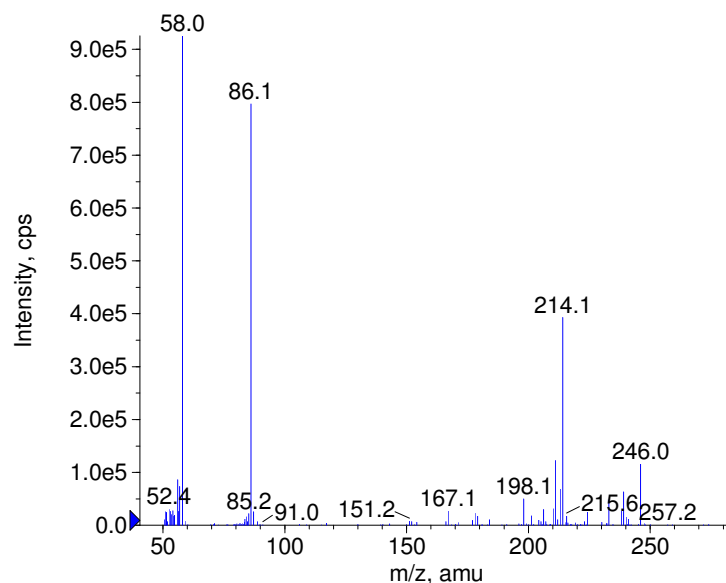
■ + Chlorpromazine Prec(319.0) CE(50.0) RT(0.8)
