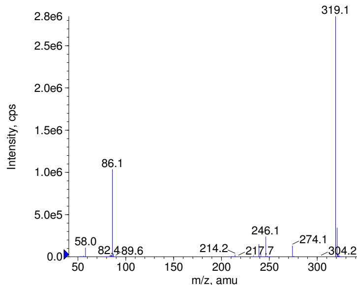
■ + Chlorpromazine Prec(319.0) CE(50.0) RT(0.8)
