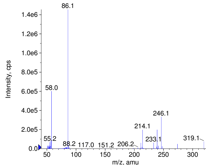
■ + Chlorpromazine Prec(319.0) CE(99.0) RT(0.8)
