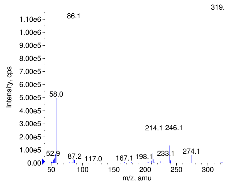
■ + Chlorpromazine Prec(319.0) CE(99.0) RT(0.8)
