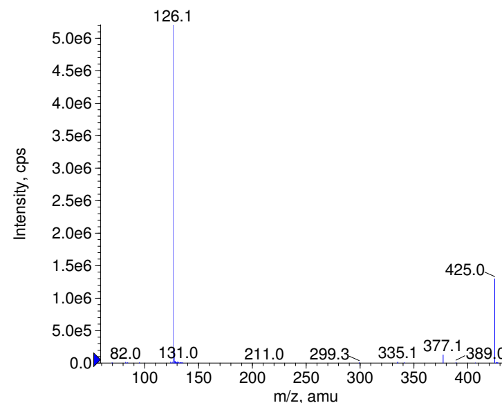
+ Clindamycin Prec(425.0) CE(99.0) RT(0.9)
