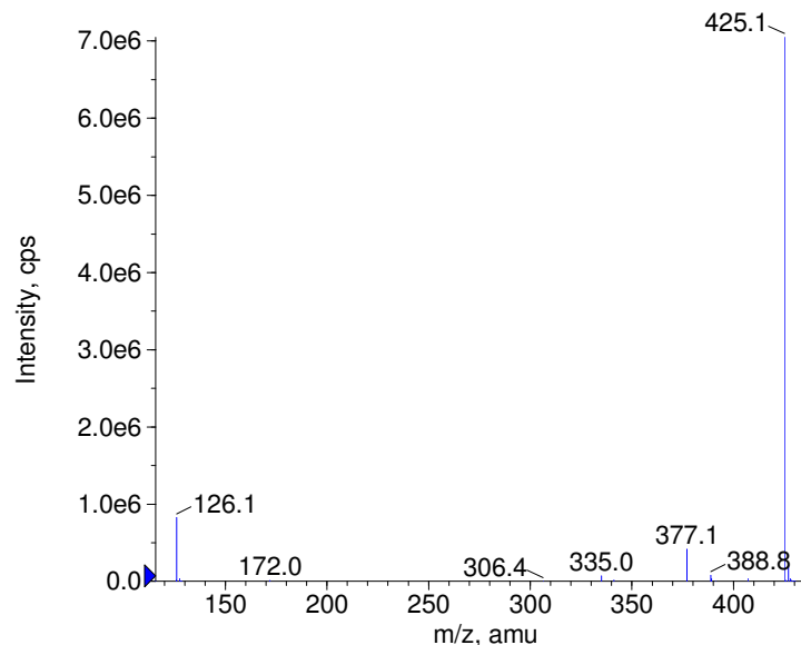
+ Clindamycin Prec(425.0) CE(50.0) RT(0.9)
