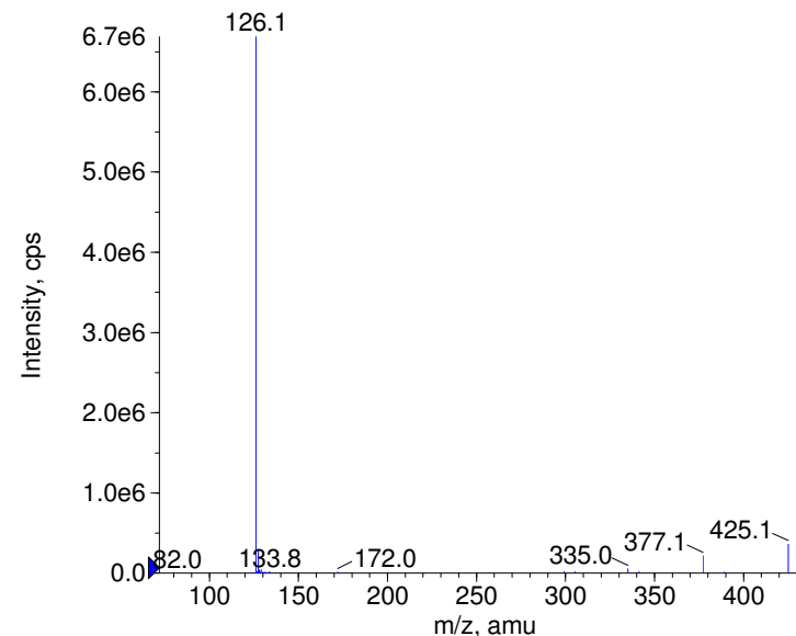
+ Clindamycin Prec(425.0) CE(99.0) RT(0.9)
