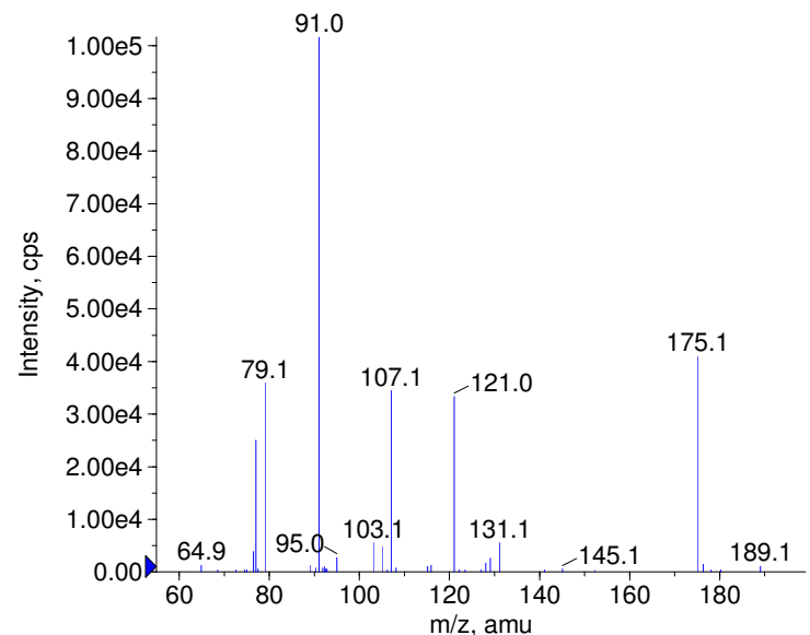
+ Coumatetralyl Prec(293.0) CE(50.0) RT(1.2)
