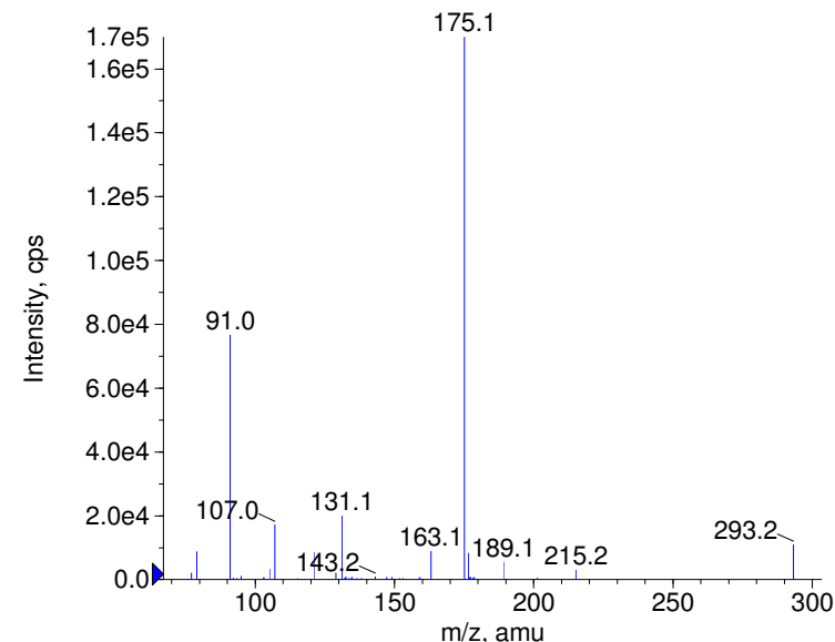
+ Coumatetralyl Prec(293.0) CE(99.0) RT(1.3)
