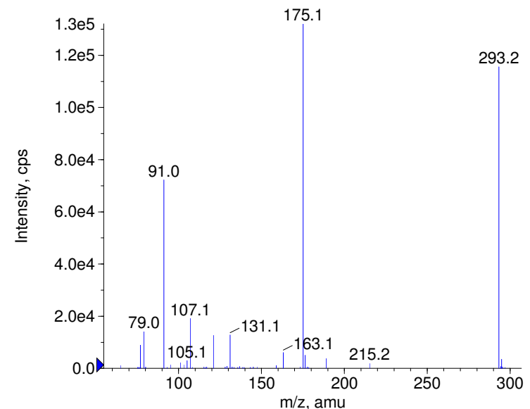
+ Coumatetralyl Prec(293.0) CE(99.0) RT(1.3)
