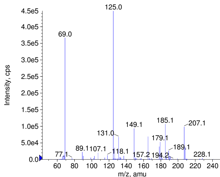
■ + Croconazole Prec(311.0) CE(50.0) RT(0.9)
