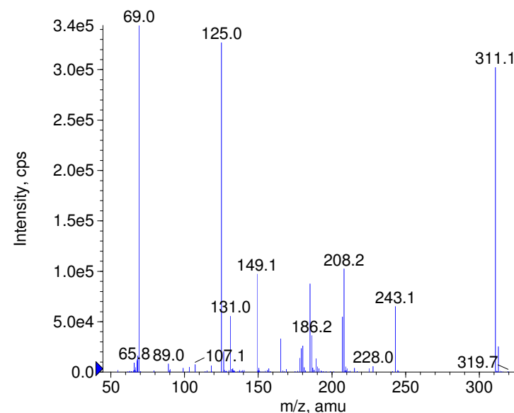
■ + Croconazole Prec(311.0) CE(99.0) RT(1.0)
