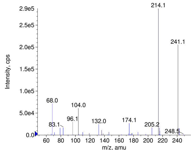
■ + Cyanazine Prec(241.0) CE(99.0) RT(0.9)
