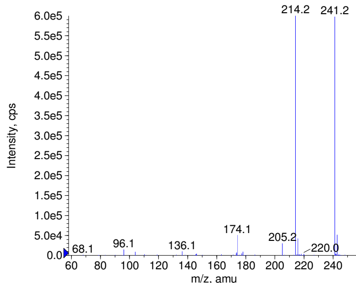
■ + Cyanazine Prec(241.0) CE(50.0) RT(0.9)
