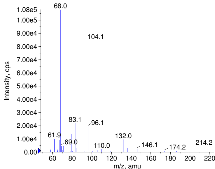
■ + Cyanazine Prec(241.0) CE(50.0) RT(0.9)
