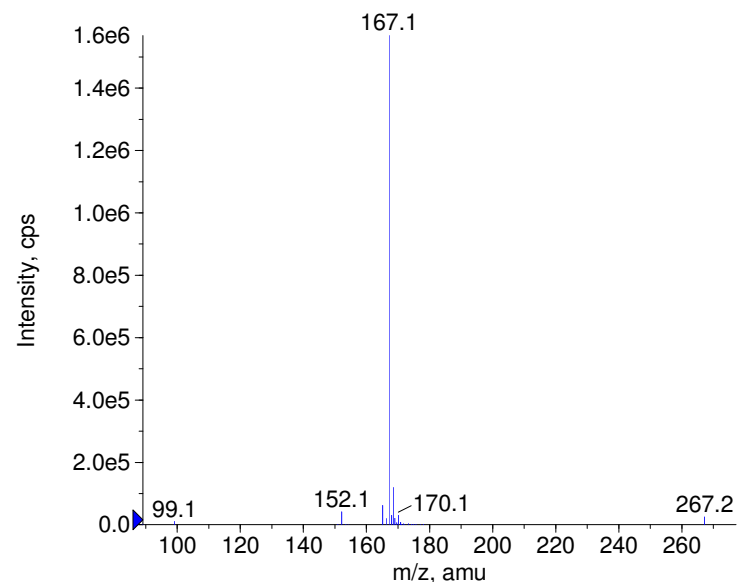
+ Cyclicine Prec(267.0) CE(50.0) RT(0.7)
