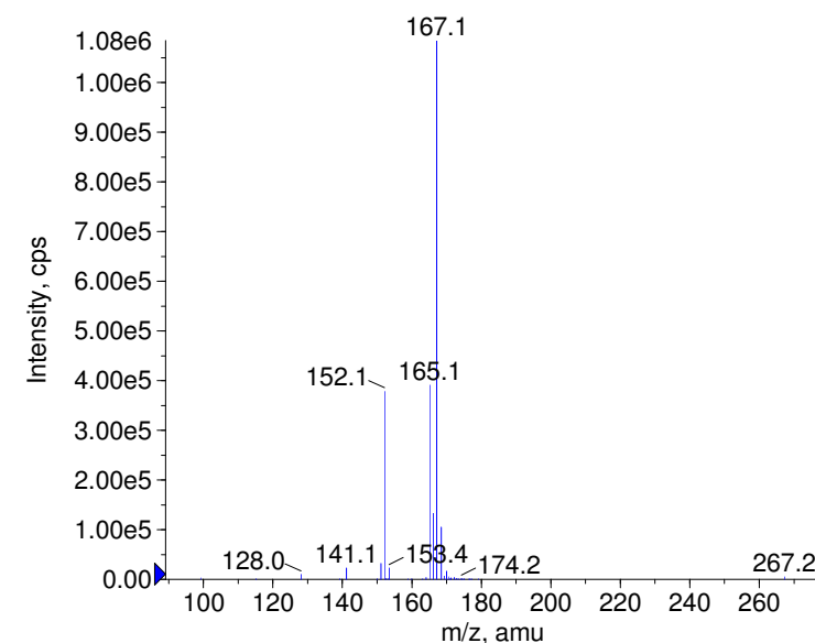
+ Cyclicine Prec(267.0) CE(99.0) RT(0.7)
