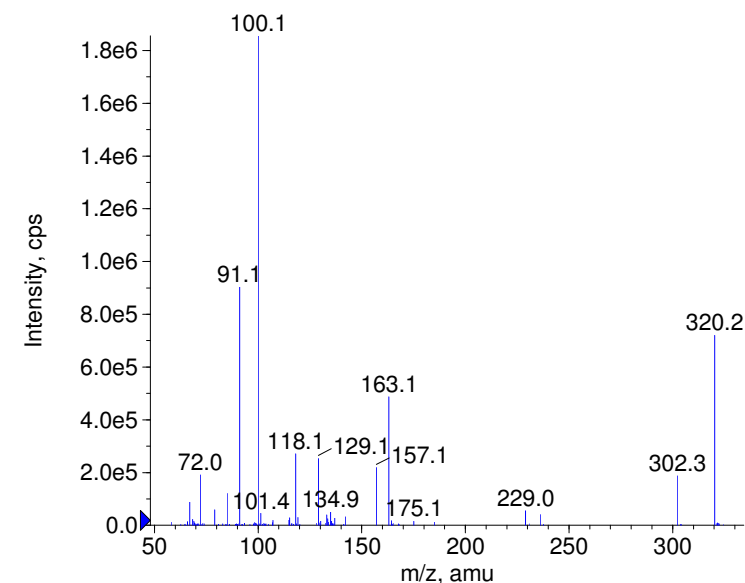
+ Cyclodrine Prec(320.0) CE(99.0) RT(0.9)
