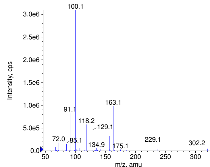
+ Cyclodrine Prec(320.0) CE(99.0) RT(0.9)
