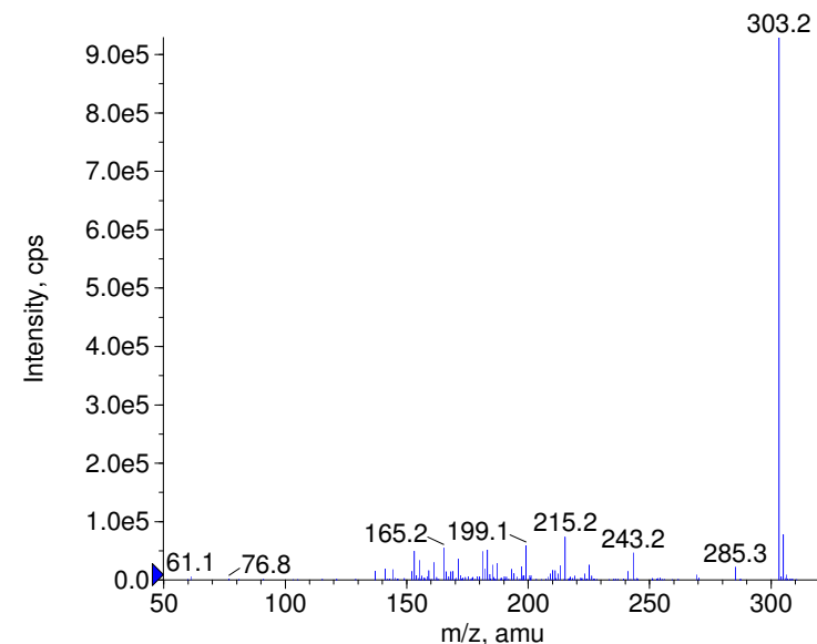
+ D3-Codeine Prec(303.0) CE(99.0) RT(0.8)
