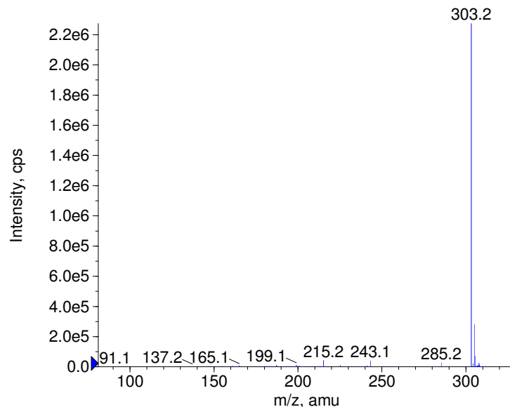
+ D3-Codeine Prec(303.0) CE(50.0) RT(0.8)
