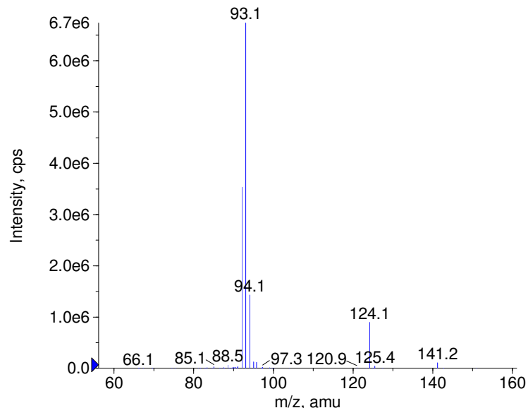
+ D5-Amphetamin Prec(141.0) CE(50.0) RT(0.8)
