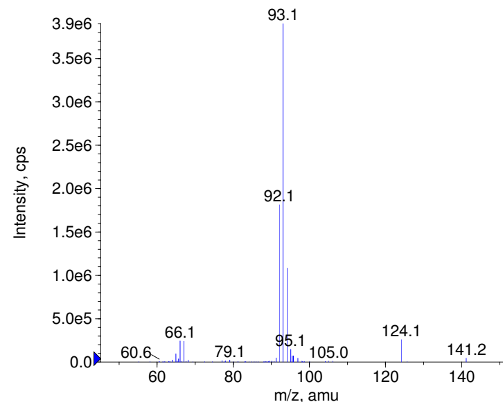
+ D5-Amphetamin Prec(141.0) CE(99.0) RT(0.9)
