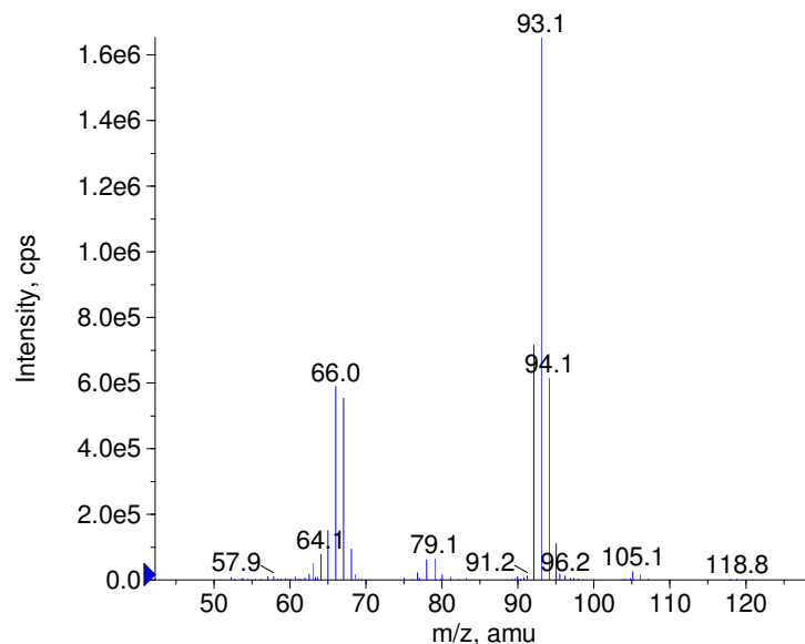
+ D5-Amphetamin Prec(141.0) CE(50.0) RT(0.8)
