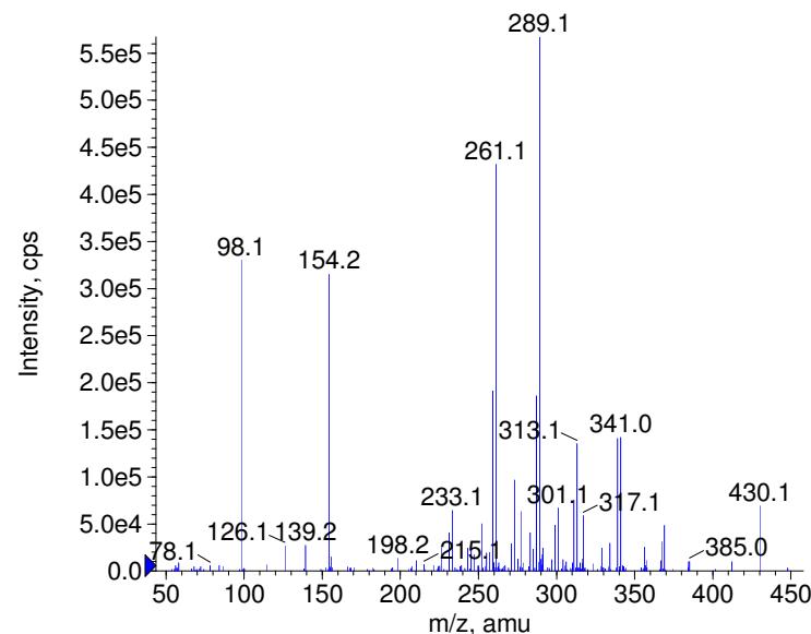
+ Demeclocycline Prec(465.0) CE(50.0) RT(1.1)
