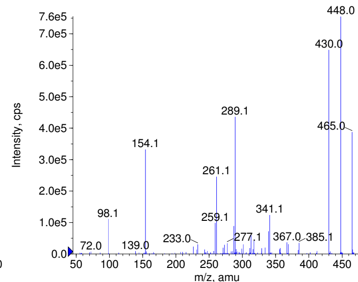
+ Demeclocycline Prec(465.0) CE(99.0) RT(1.1)
