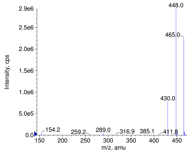
+ Demeclocycline Prec(465.0) CE(50.0) RT(1.1)
