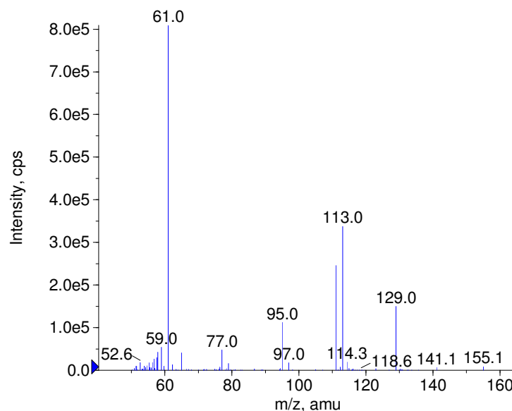
+ Demeton-O-methyl Prec(231.0) CE(50.0) RT(0.8)
