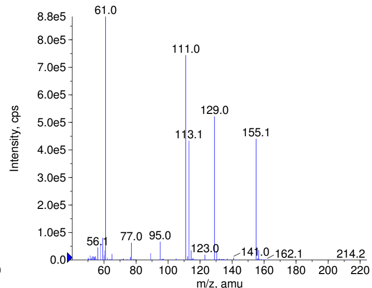
+ Demeton-O-methyl Prec(231.0) CE(99.0) RT(0.9)
