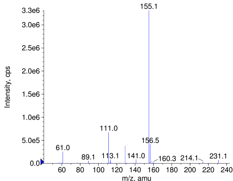
+ Demeton-O-methyl Prec(231.0) CE(50.0) RT(0.8)
