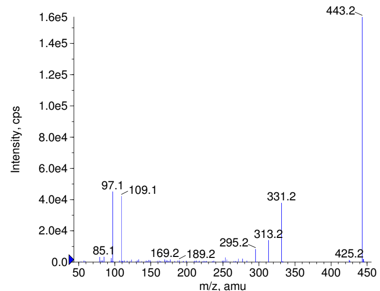
+ Desoxycortone enantate Prec(443.0) CE(99.0) RT(5.5)
