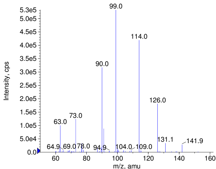
+ Diazoxide Prec(231.0) CE(50.0) RT(1.0)
