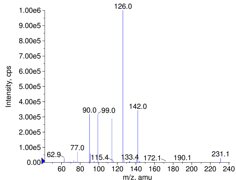
+ Diazoxide Prec(231.0) CE(99.0) RT(1.0)
