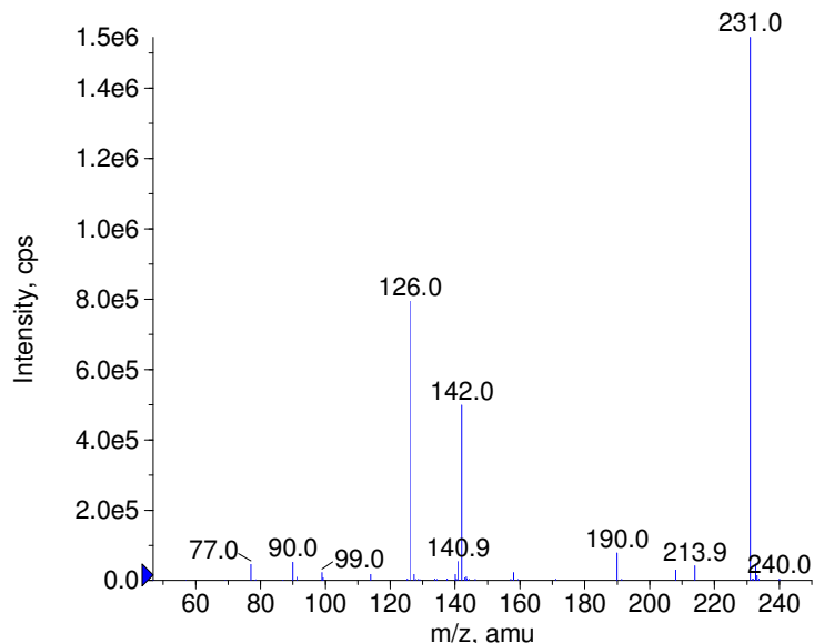
+ Diazoxide Prec(231.0) CE(50.0) RT(1.0)
