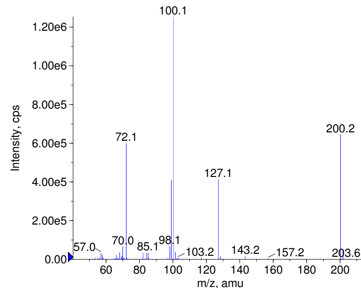
+ Diethylcarbamazine Prec(200.0) CE(99.0) RT(0.8)
