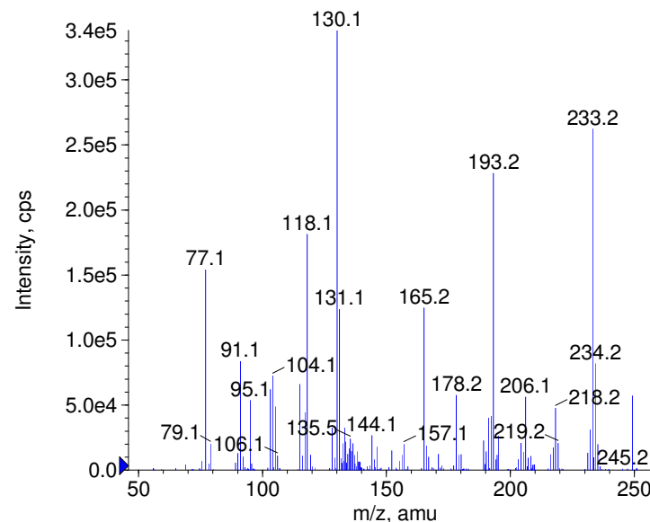
+ Difenzoquat Prec(249.0) CE(50.0) RT(0.8)
