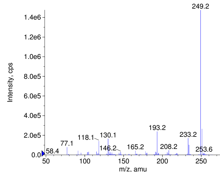
+ Difenzoquat Prec(249.0) CE(99.0) RT(0.8)
