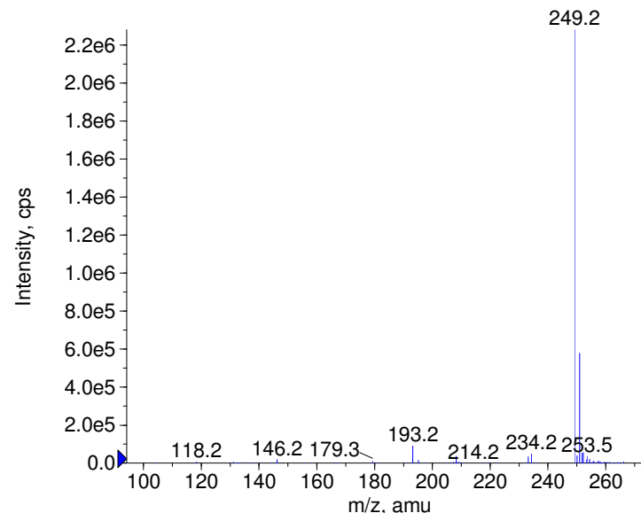
+ Difenzoquat Prec(249.0) CE(50.0) RT(0.8)
