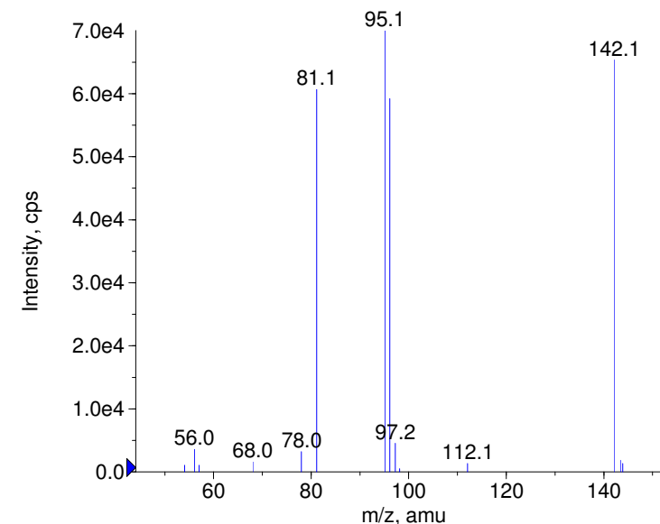
+ Dimetridazole Prec(142.0) CE(99.0) RT(0.9)
