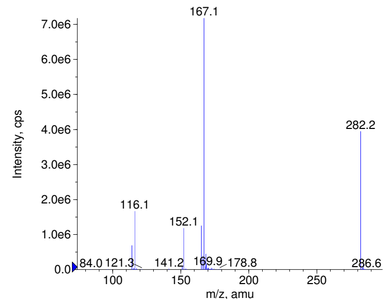
+ Diphenylpyraline Prec(282.0) CE(99.0) RT(0.9)
