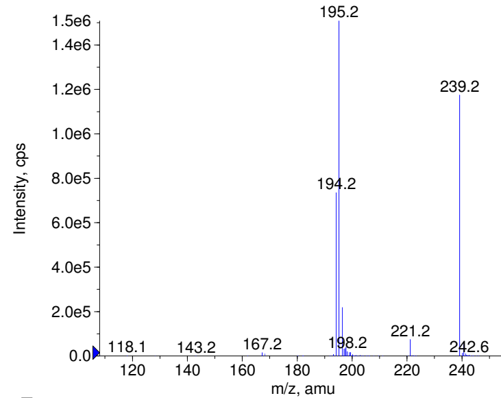
■ + Disopyramide Prec(340.0) CE(99.0) RT(0.8)
