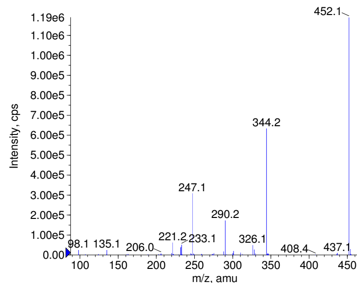
+ Doxazosin Prec(452.0) CE(99.0) RT(1.0)
