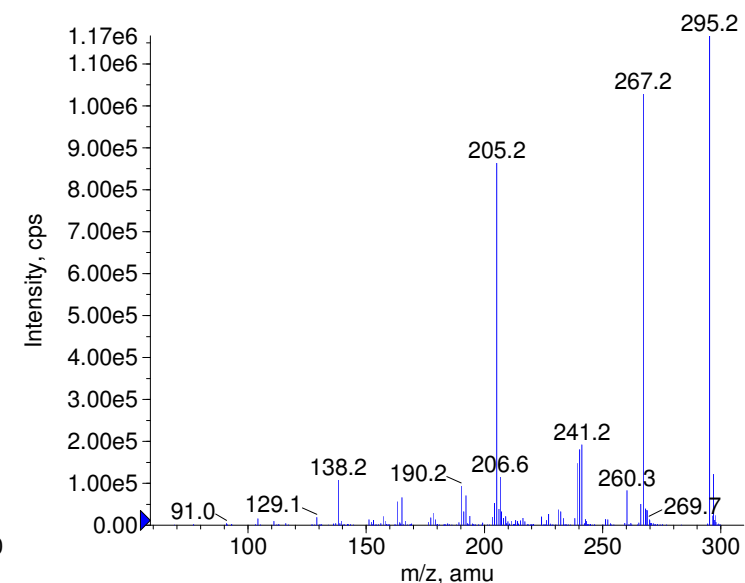
+ Estazolam Prec(295.0) CE(99.0) RT(0.8)
