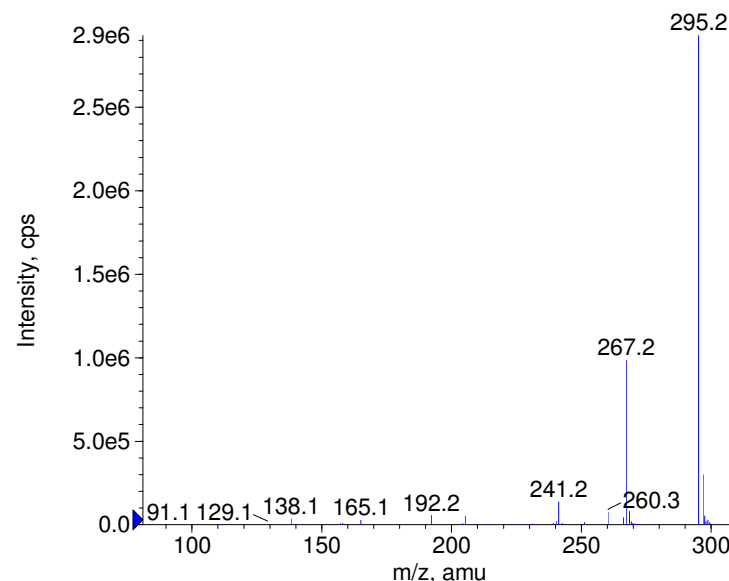
+ Estazolam Prec(295.0) CE(50.0) RT(0.8)
