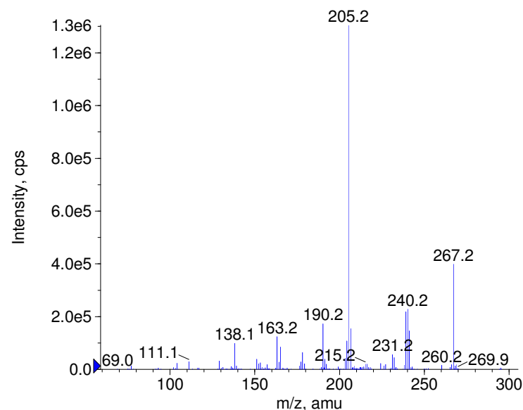
+ Estazolam Prec(295.0) CE(50.0) RT(0.8)
