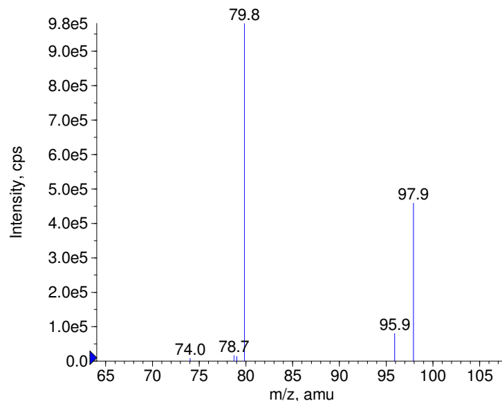
■ - Ethyl sulfate-D5 Prec(130.0) CE(-50.0) RT(0.8)
