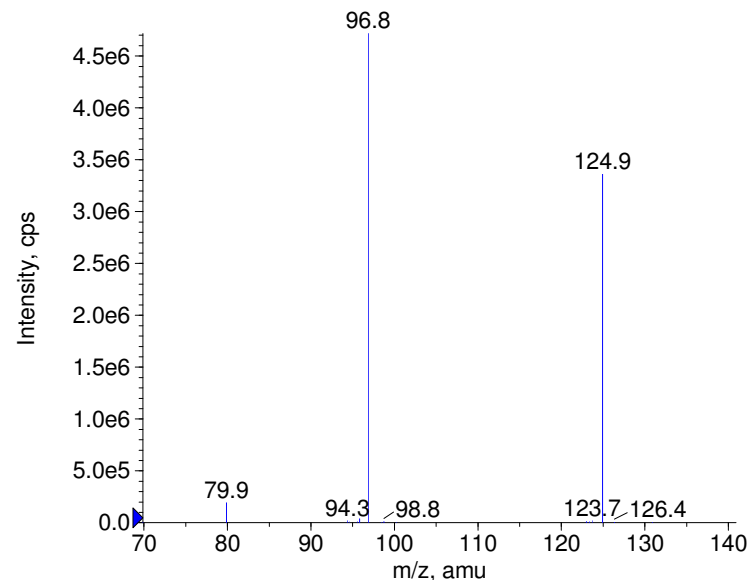
■ - Ethyl sulfate Prec(125.0) CE(-50.0) RT(1.0)
