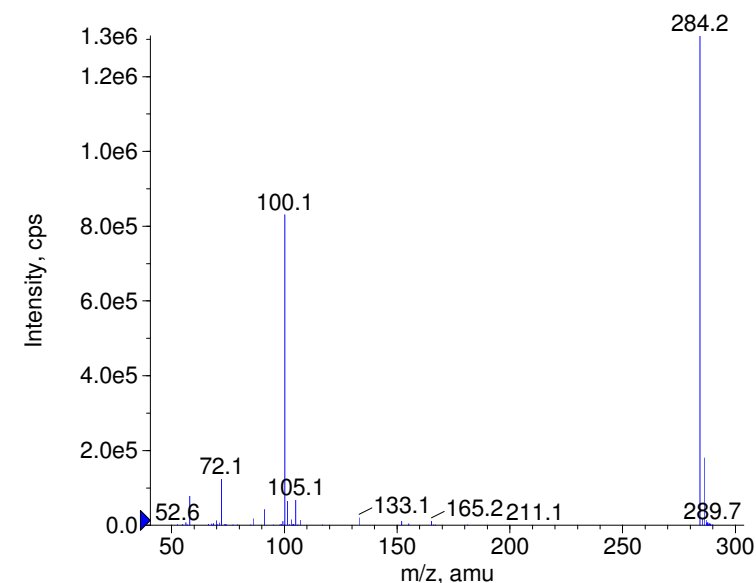
+ Etoloxamine Prec(284.0) CE(99.0) RT(0.9)
