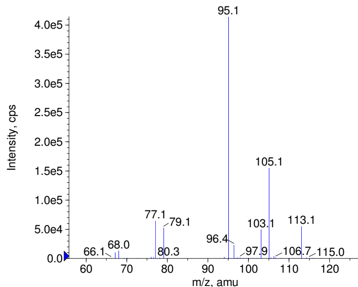
■ + Etomidate Prec(245.0) CE(50.0) RT(1.0)
