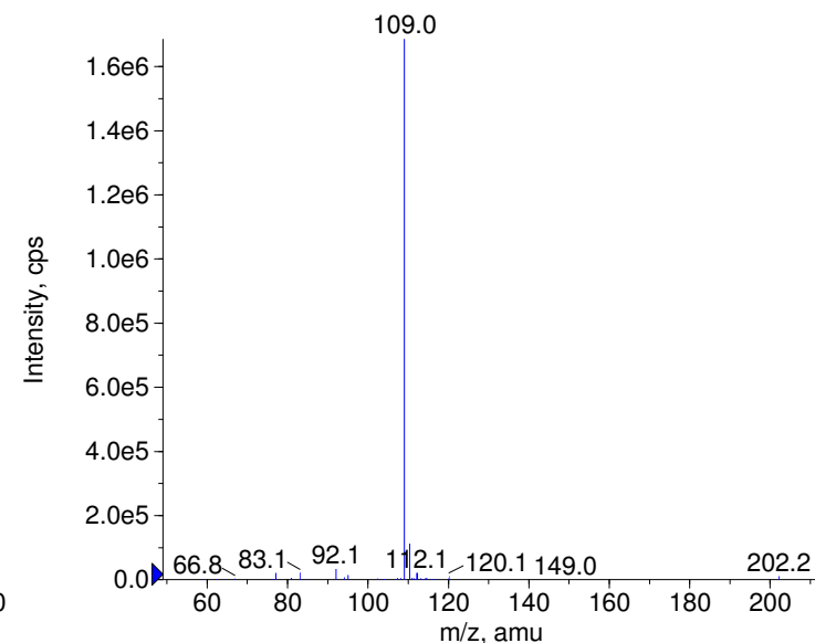
+ Fenfuram Prec(202.0) CE(99.0) RT(1.0)
