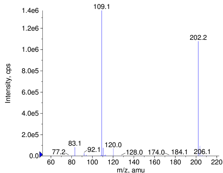
+ Fenfuram Prec(202.0) CE(50.0) RT(1.0)
