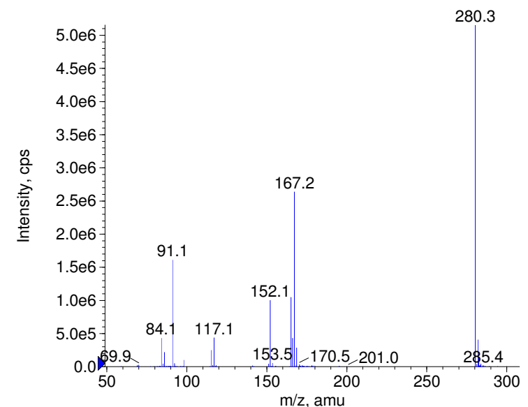
+ Fenpiprane Prec(280.0) CE(99.0) RT(0.8)
