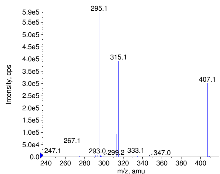
■ + Floctafenine Prec(407.0) CE(99.0) RT(1.0)
