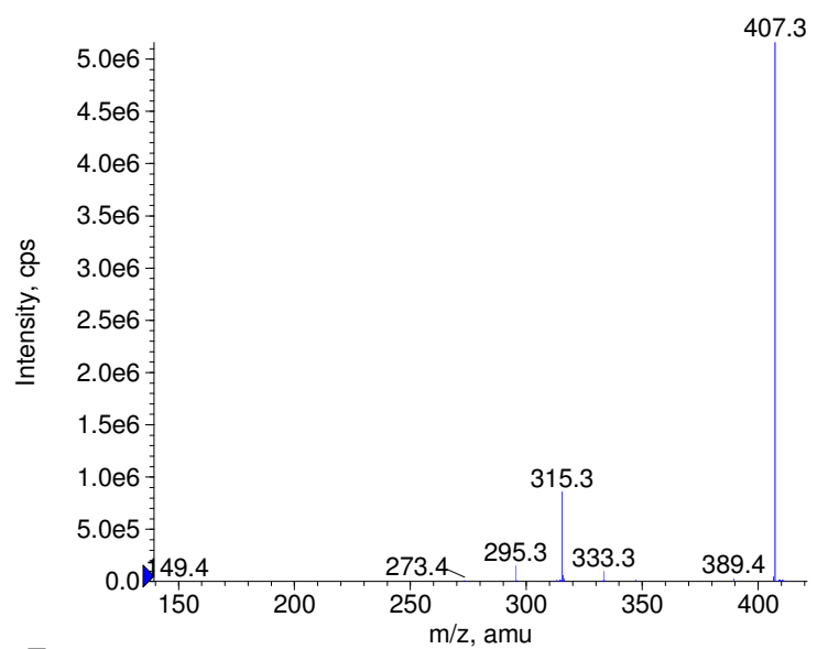
■ + Floctafenine Prec(407.0) CE(50.0) RT(1.0)
