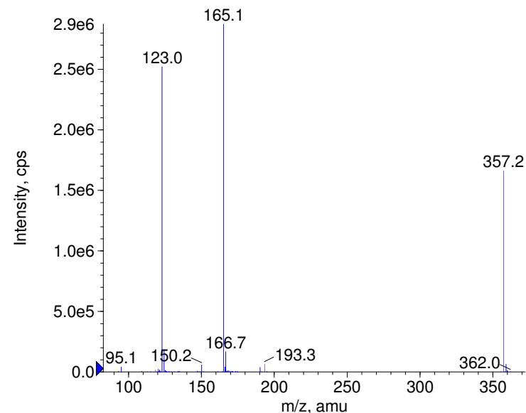
+ Fluanisone Prec(357.0) CE(99.0) RT(0.9)
