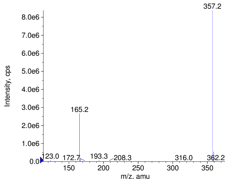
+ Fluanisone Prec(357.0) CE(50.0) RT(0.9)
