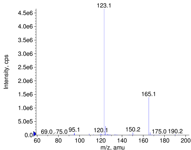
+ Fluanisone Prec(357.0) CE(50.0) RT(0.9)
