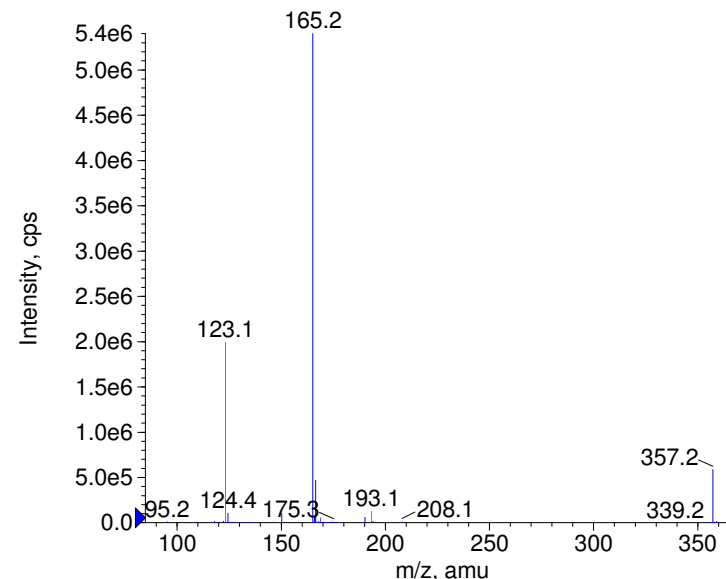
+ Fluanisone Prec(357.0) CE(99.0) RT(0.9)
